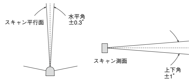
(図-2 機械軸と光軸のずれ)
